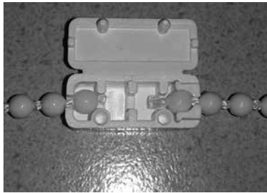
Ausführung kindersicher: mit Abreißsystem von 6 kg innerhalb von 5 s. Verbindung mit 1 Kugel
